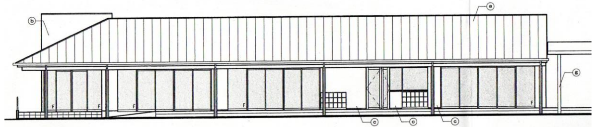
東面
