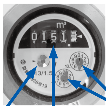
パイロット カウンター(m³) 赤い針(ℓ)
